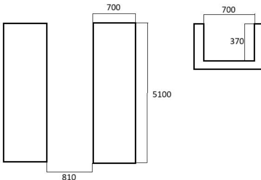
Ryc.1. Schemat i wymiary miejsca osadzenia urządzenia
