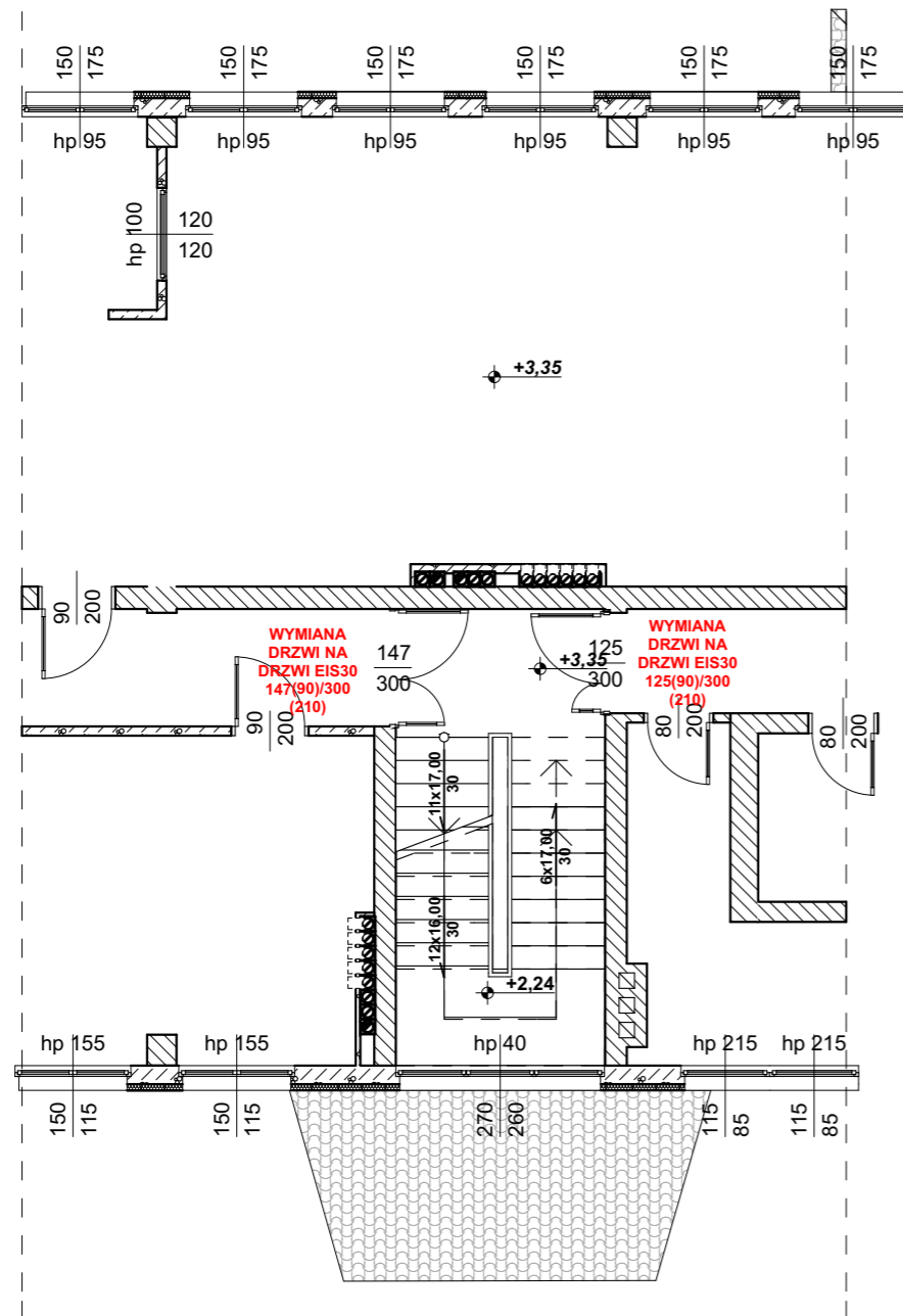
RZUT I PIĘTRA
